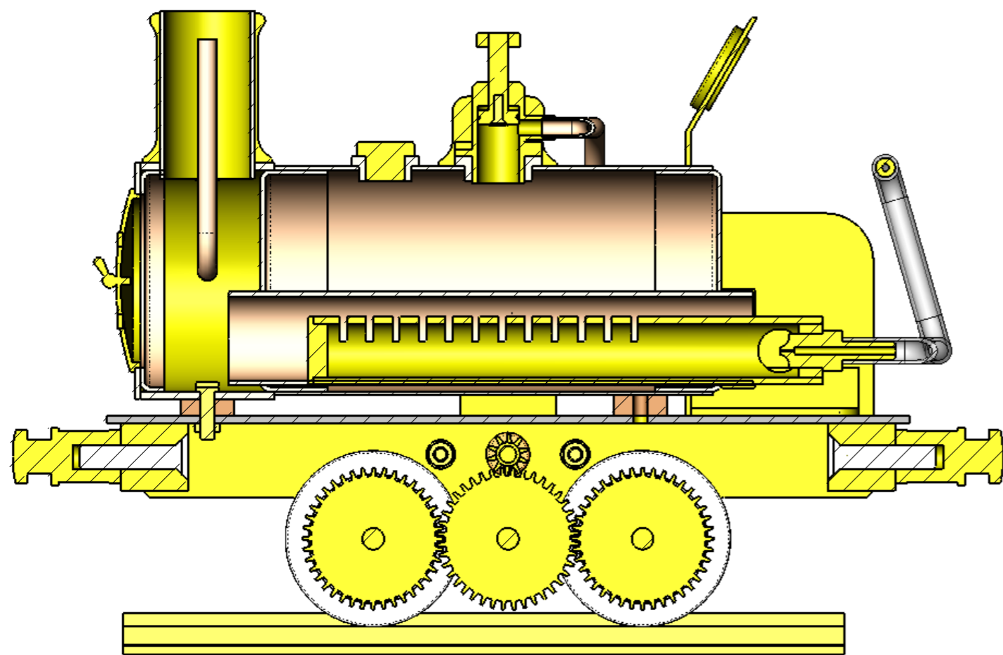
SECTION A-A SCALE 1 : 1.1
